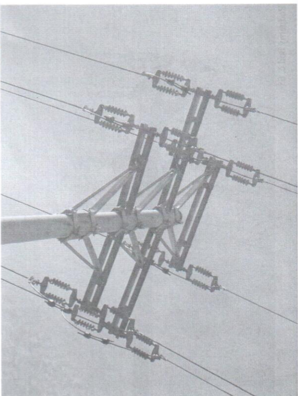
Podperný bod č. 64
