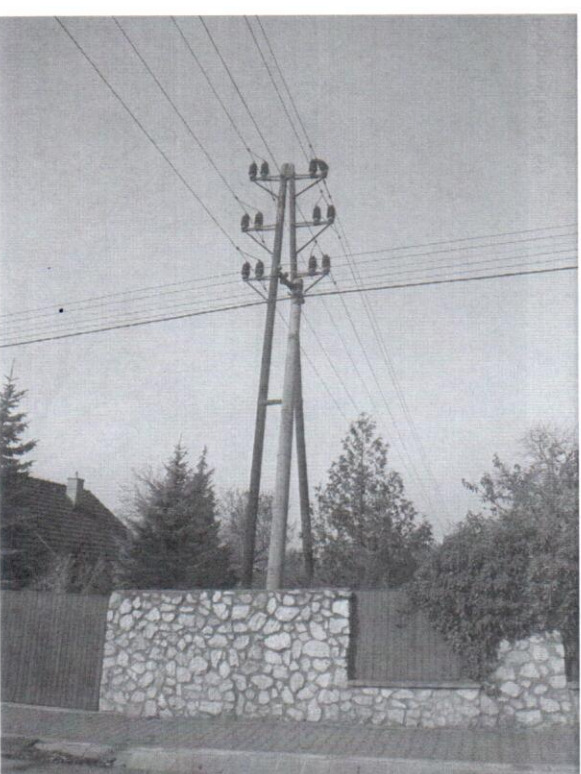
Križenie s NN VSE (VO) Rozhlas na Bysstrickej ulici a Podperný bod č. 66
